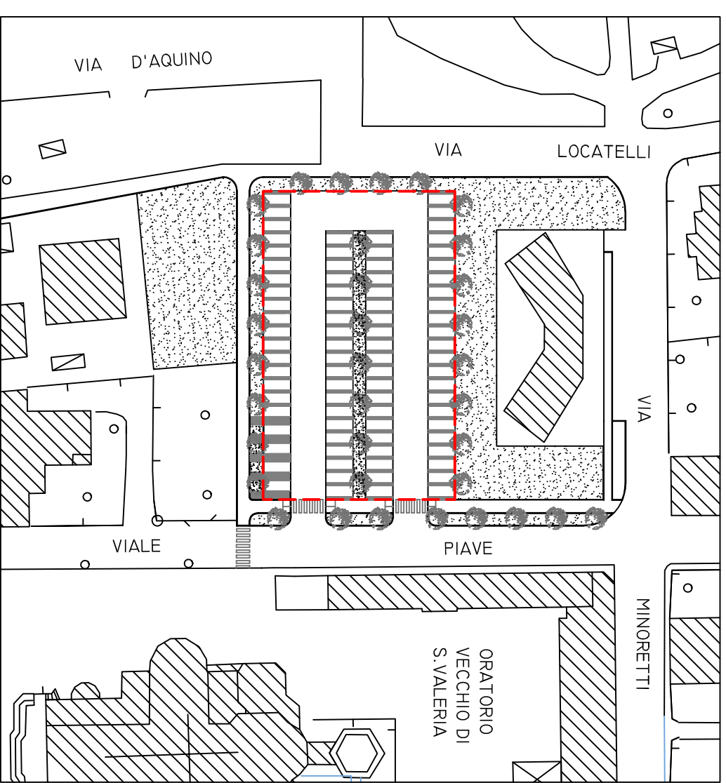
aerofotogrammetrico scala 1:1000
